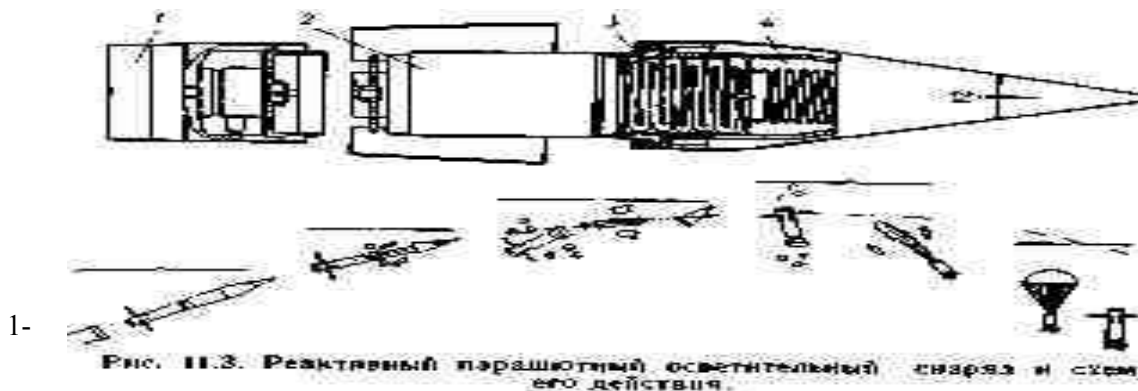
Рис. 11.3. Реактивный парашютный осветительный снаряд и схем. его действия
