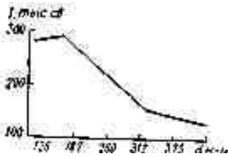
Рис. 11. 12. Зависимость силы света состава (Mg+NaN03+ 4-поливинилхлорид+смола) от размера частиц магния
