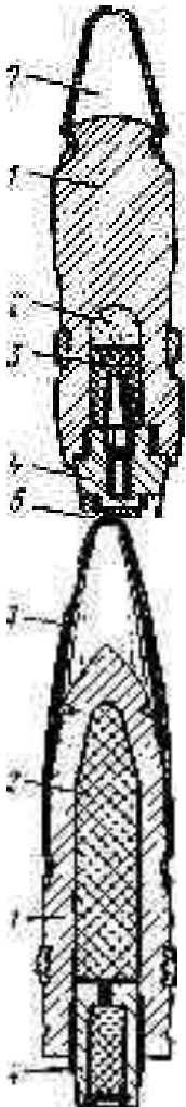
Рис. 15.6. Бронебой-но-зажигательно-трассирующий снаряд'
