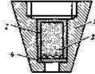
Рис. 13.7. Трассер к взрывателю МД-5:
