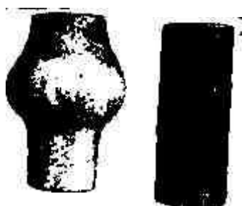
Рис 9.2 Толстостенный свинцовый цилиндр до (слева) и после взрыва в нем 50 г стехиометрической смеси H 2 O+Mg, инициатор — капсюль-детонатор № 8
