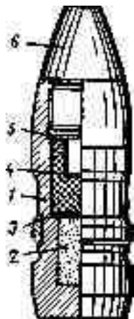
Рис. 15.1. Осколочно-зажигательный снаряд:
