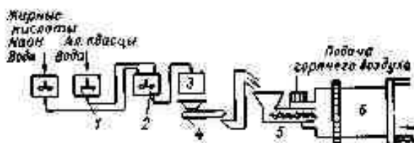
Рис. 15.12. Схема получения напалмового загустителя:
