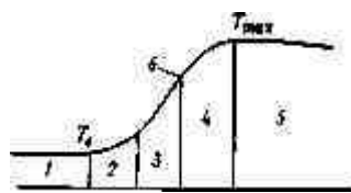
Рис. 8.1. Схема горения пиротехнического состава: 1-пиротехнический состав; 2-зона прогрева; 3-зона реакции в конденсированной фазе; 4-зона реакции в газовой фазе; 5-продукты реакции; 6- реакция на поверхности раздела фаз
