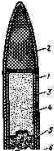
Рис. 13.1. Трассирующая пуля Т-30 образца 1930 г.:
