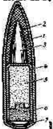
Рис. 13.2. Бронебойно-трассирующая пуля БТ-32:
