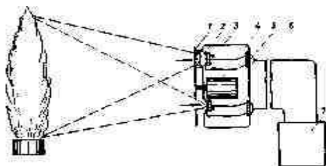
Рис. 6.2. Схема цветного пирометра: 1-вращающийся диск; 2-светофильтр; 3-фотоэлемент; 4-электродвигатель; 5-выводы контактов; 6-корпус; 7—осциллограф
