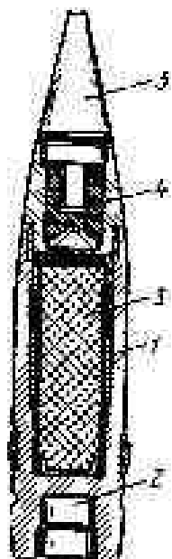
Рис. 15.2. Осколочно-зажигательно - трассирующий снаряд (патент ФРГ 1.278.290, 1968 г.):
