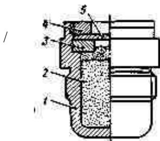
Рис. 13.5. Трассер:
