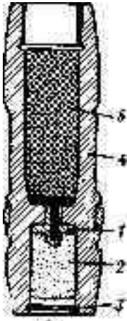
Рис. 13.10. Осколочно-зажигательно - трассирующий зенитный снаряд с самоликвидацией через трассер:
