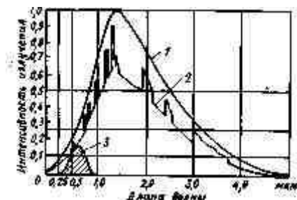
Рис. 11.8. График распределения энергии по спектру: 1—АЧТ при 3000 К; 2—осветительный состав; 3—кривая видности человеческого глаза
