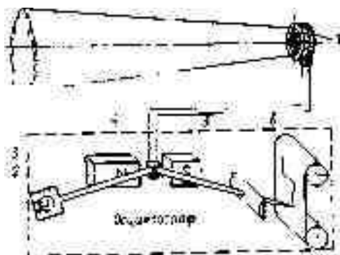
Рис. 11.20. Схема измерения силы света: 1—светоприемник; 2—осветитель; 3—диафрагма; 4—шлейф; 5—цилиндрическая линза; 6—фотобумага
