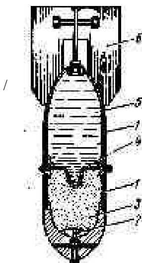
Рис. 15.11. Бомба комбинированного снаряжения ЗАБ-80-ТГ [17]: — корпус; 2—воспламеняющая шашка; 3— термитно-зажигательный состав; 4—диафрагма; 5—отвержденное горючее; 6— стабилизатор
