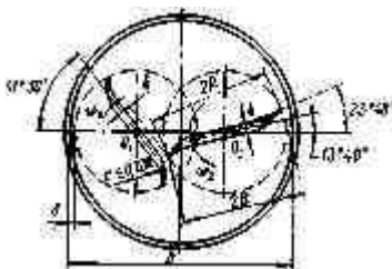
Рис. 22.5. Размеры чаши смесителя .
