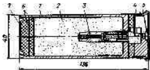
Рис. 12.9. Устройство типичного фотопатрона: 1— оболочка фотозаряда; 2— фотосмесь; 3— замедлительно-воспламенительное устройство (ЗВУ); 4— вышибной пороховой заряд; 5— капсюльная втулка; 6— пыжи фотозаряда; 7— крышка патрона
