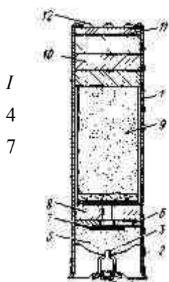
Рис. 11.5. 26-мм осветительный патрон :
