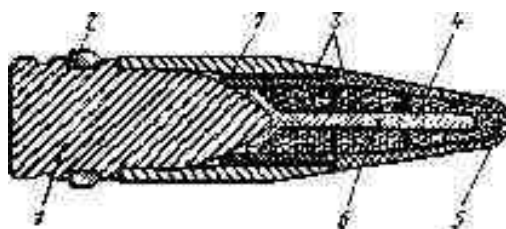
Рис. 15.3. Американский 20-
