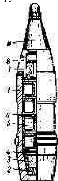
Рис. 15.8. Артиллерийский сегментный снаряд рассеивающего действия: 1—корпус; 2—донный вкладыш; 3—вышибной заряд; 4—диафрагма; 5—зажигательный сегмент; 6—прокладка; 7—головной вкладыш; 8—головка; 9— дистанционная трубка
