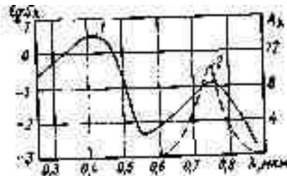
Рис. 12.4. Кривые спектральной чувствительности (Л и фотоакти-ничного потока (А)) под красным светофильтром КС-14 (2) инфра-хроматической аэрофотопленки
