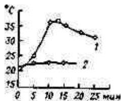
Рис. 10.1. Повышение температуры порошков магния (1) и алюминия (2) при добавлении к ним воды
